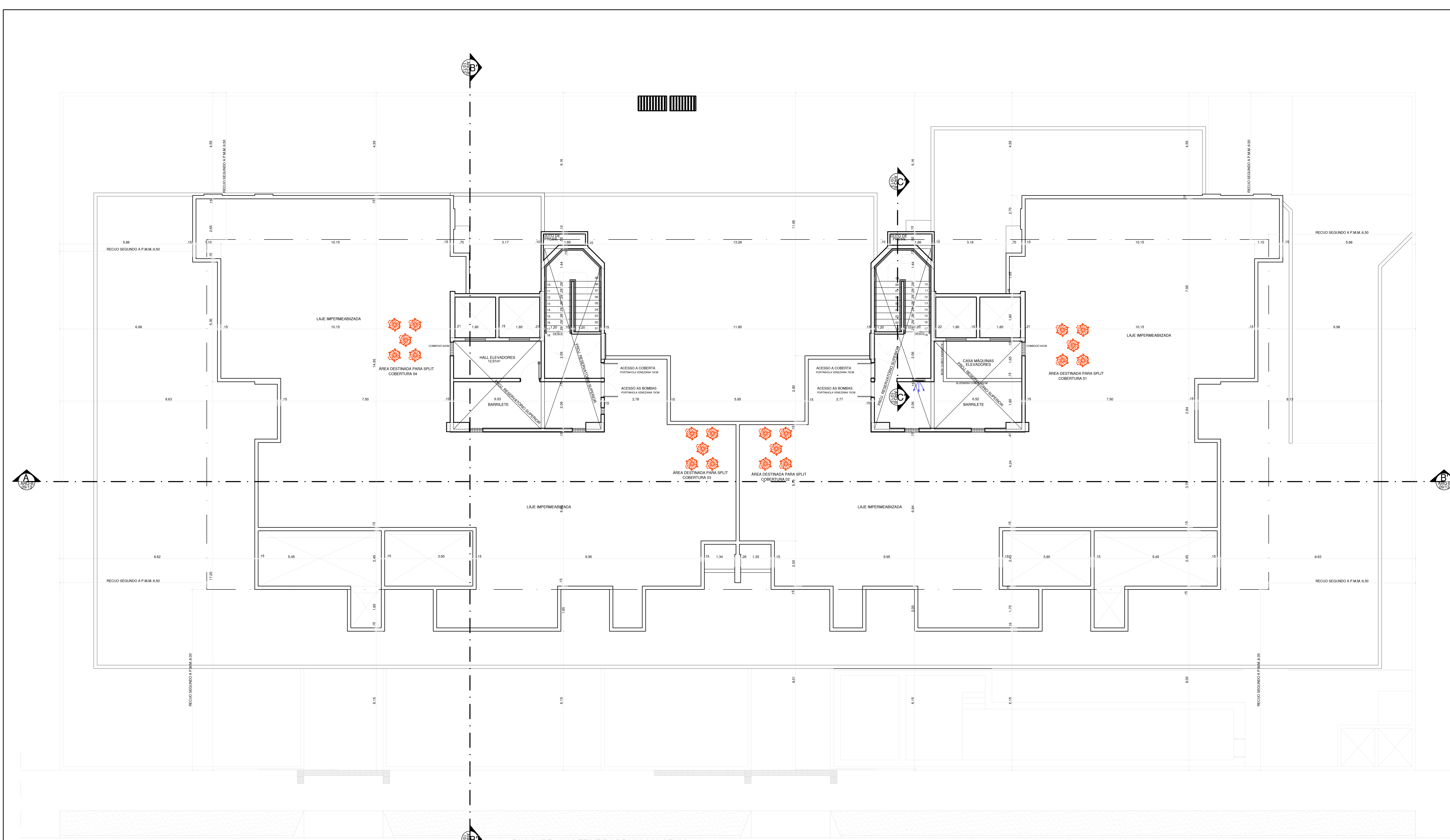
PLANTA BAIXA - ÁTICO ESC.: 1:50
