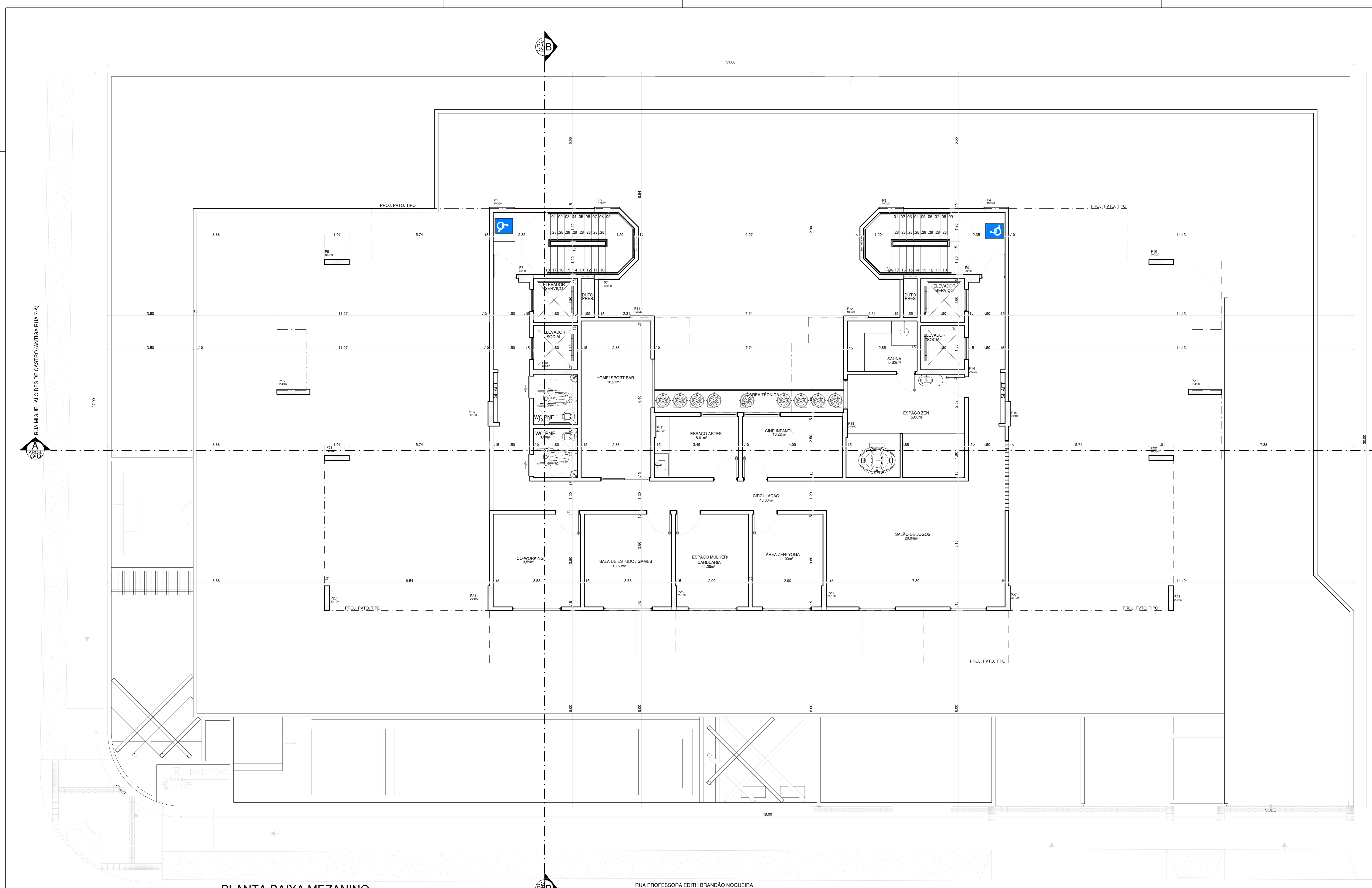
PLANTA BAIXA MEZANINO ESC. 1/50
