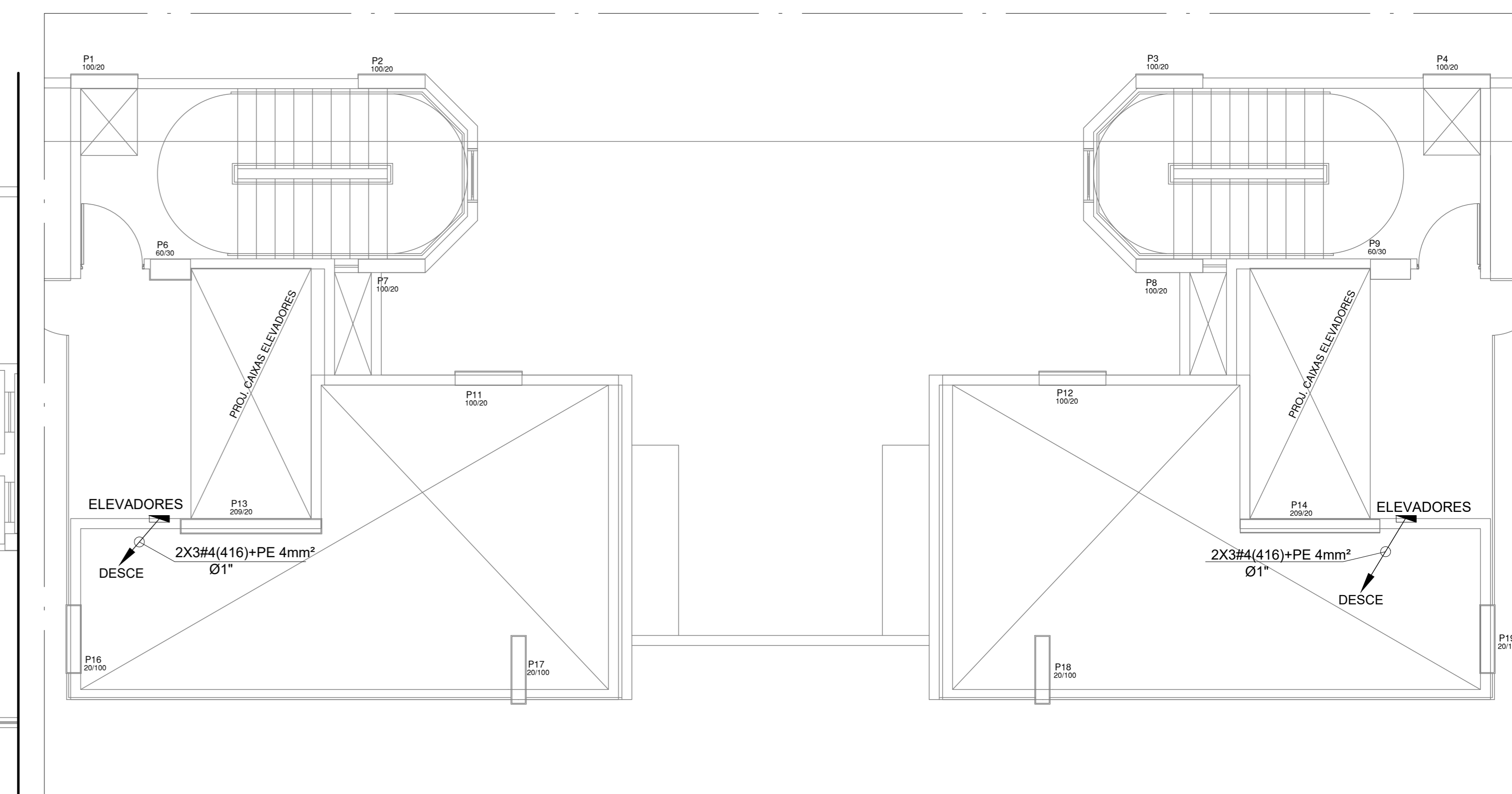
PLANTA BAIXA - ÁTICO - ALIMENTADORES ESCALA.....1/75
