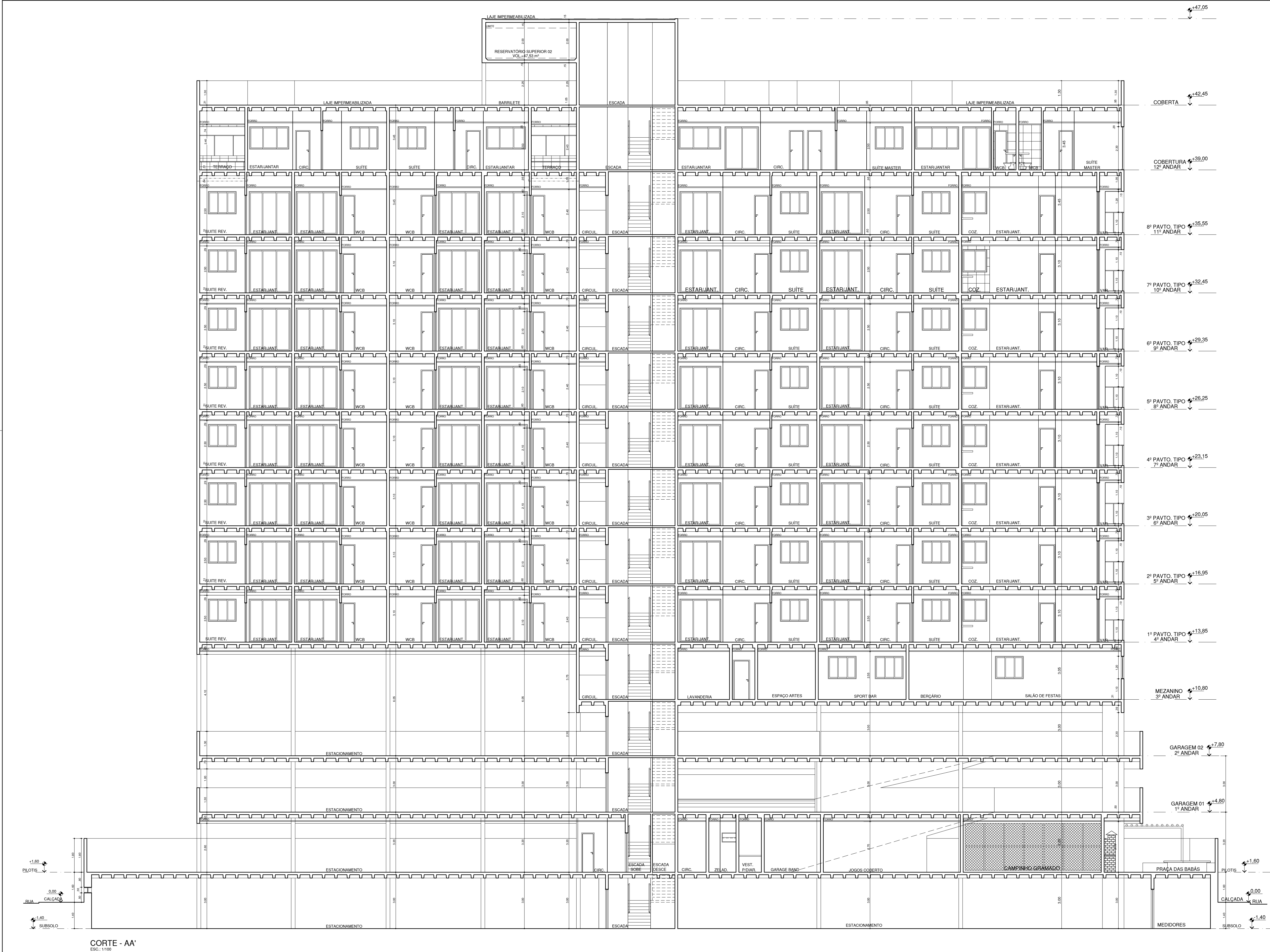
CORTE - AA'
