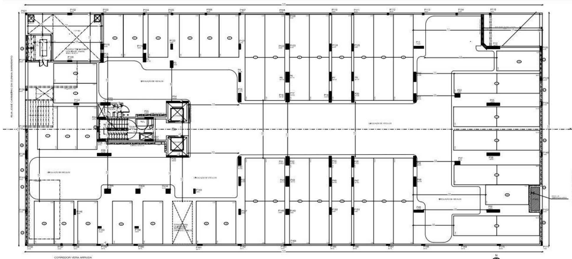
Figura 2 - Planta baixa Pavimento Subsolo
