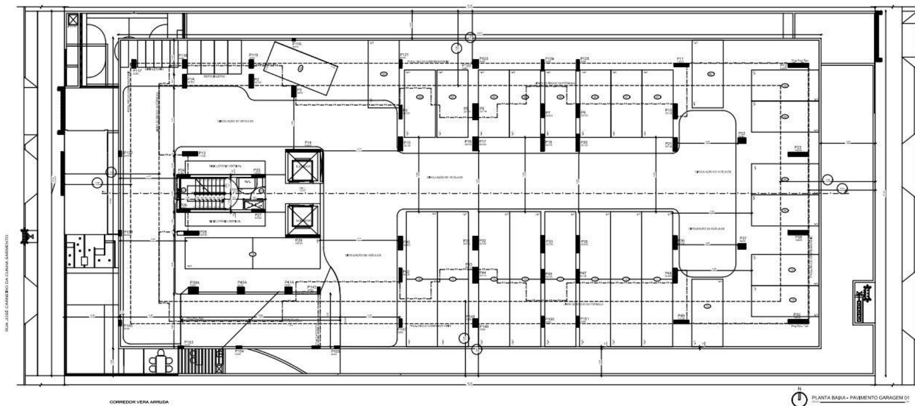
Figura 4 - Planta baixa Pavimento Garagem 01
