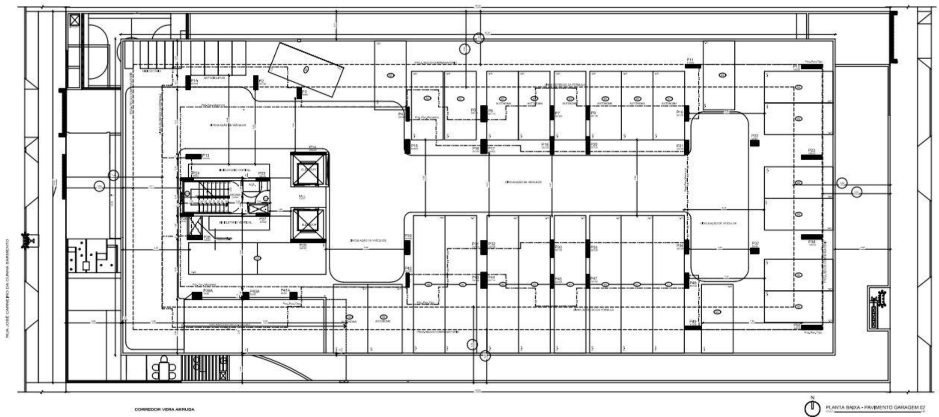
Figura 5 - Planta baixa Pavimento Garagem 02
