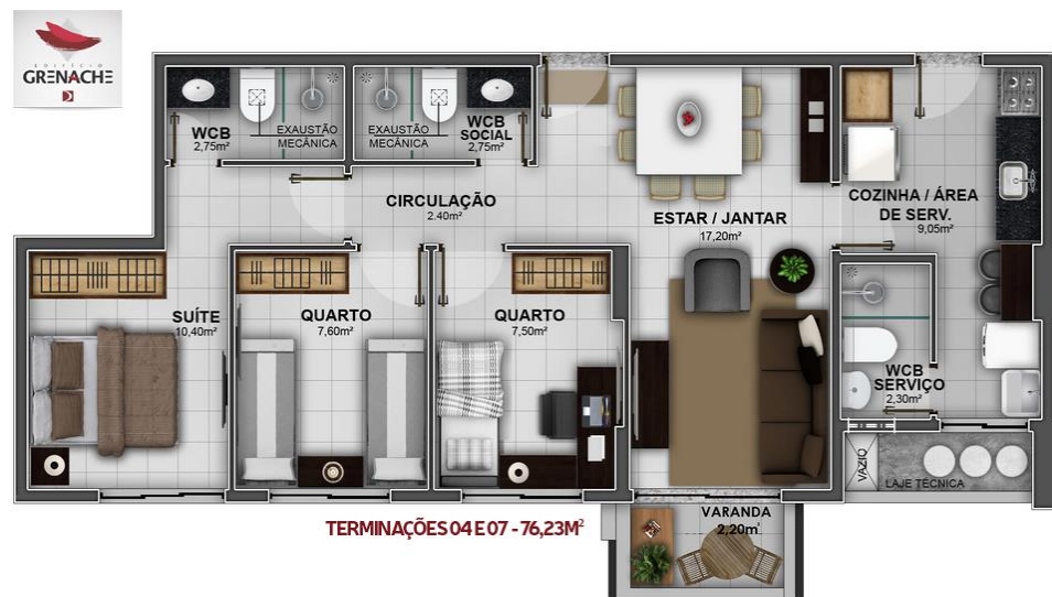
Figura 10 - Planta baixa dos Apartamentos Tipo com terminações 04 e 07
