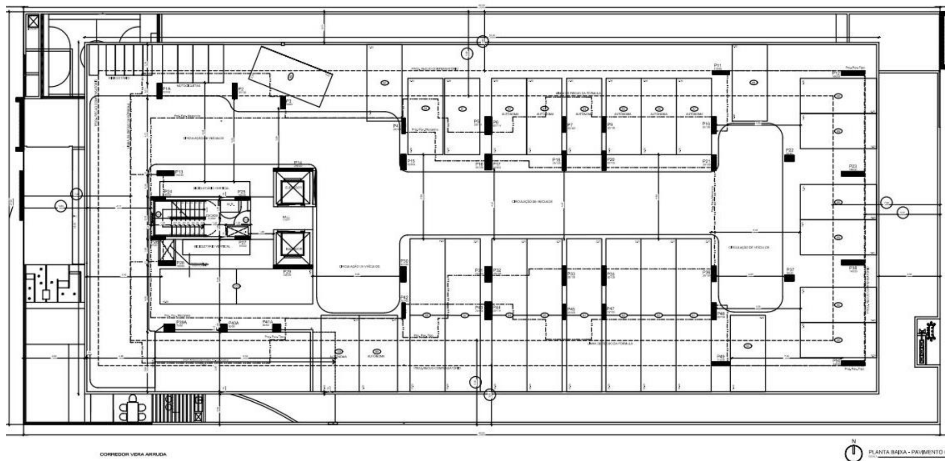
Figura 5 - Planta baixa Pavimento Garagem 02
