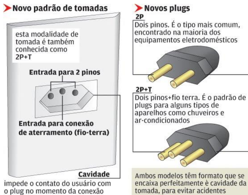
Figura 16 - Novo padrão de tomadas
