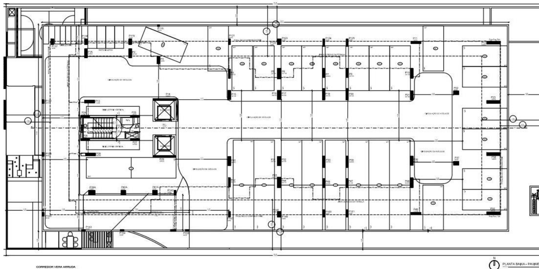
Figura 4 - Planta baixa Pavimento Garagem 01
