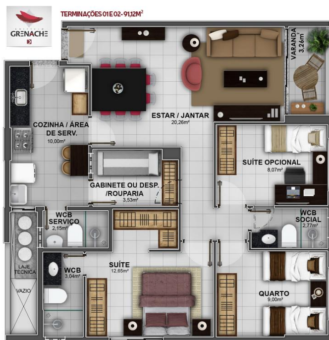
Figura 8 - Planta baixa dos Apartamentos Tipo com terminações 01 e 02
