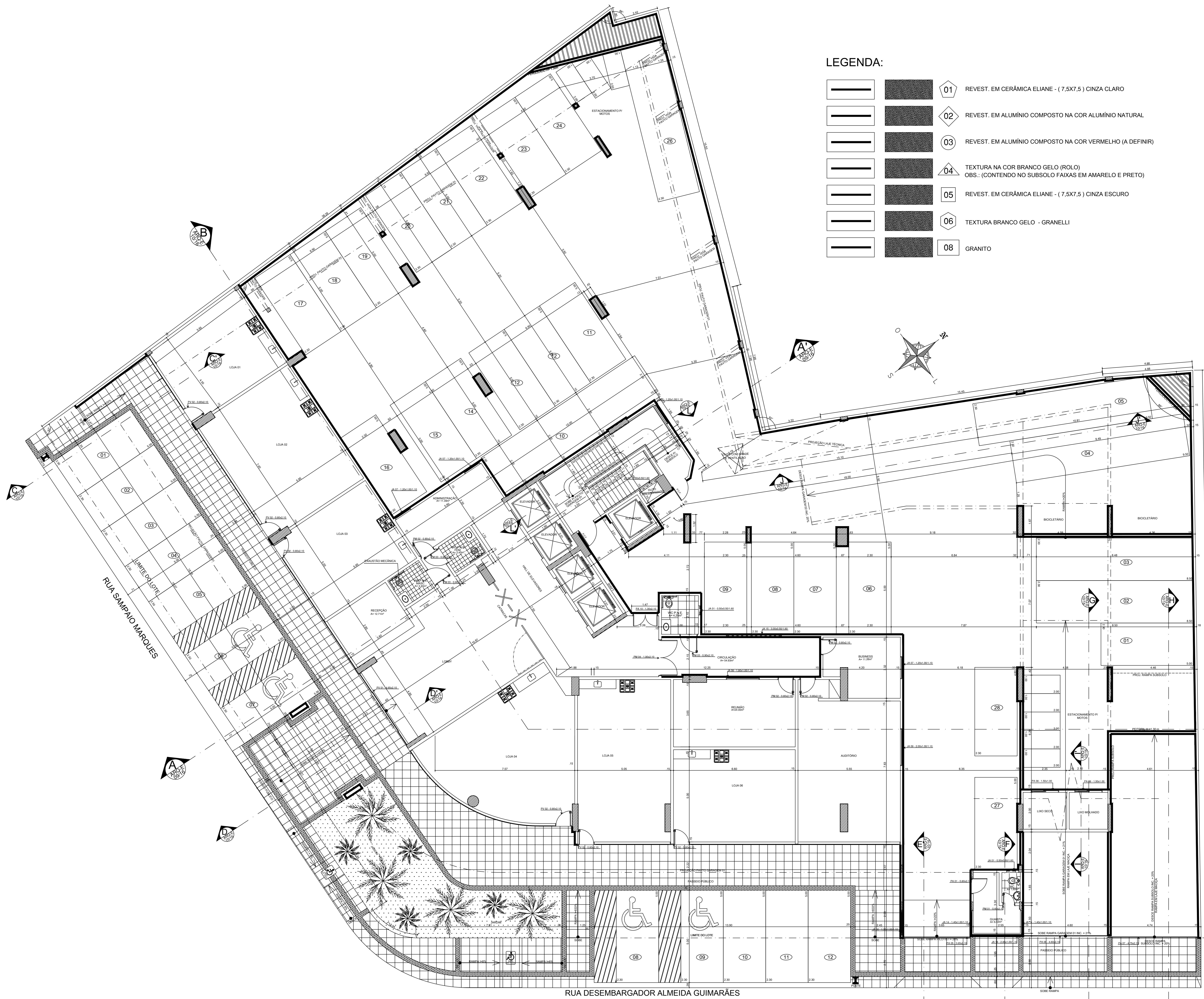
PLANTA BAIXA - PILOTIS ESC. 1/75
